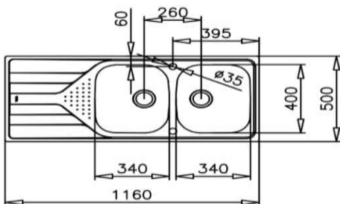
Diagrama de instalación
