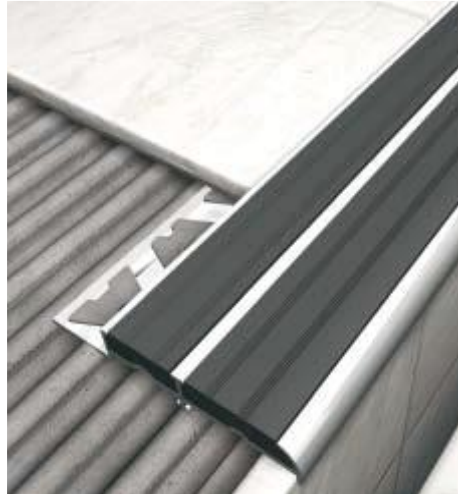
M. NARIZ ESCALON DOBLE/A67 MOL-17-0017 Nariz Escalón Doble 57x12x2500mm Aluminio/PVC Negro
