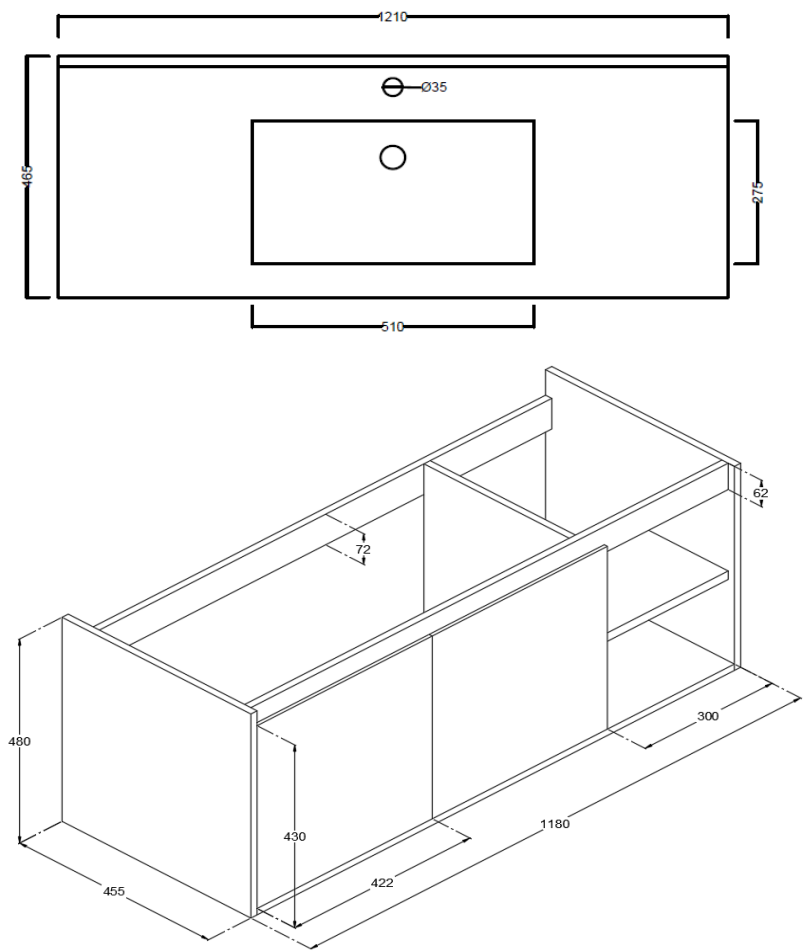
MUEBLE NEPAL 2 PUERTAS Y REPISA LATERAL 1200 MM
