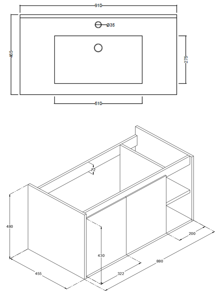
MUEBLE NEPAL 2 PUERTAS Y REPISA LATERAL 900 MM
