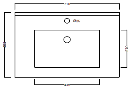
MUEBLE NEPAL 2 PUERTAS Y REPISA LATERAL 700 MM
