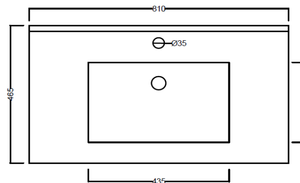
MUEBLE NEPAL 2 PUERTAS Y REPISA LATERAL 800 MM
