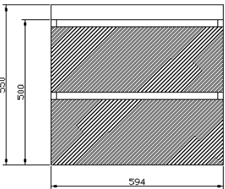
MUEBLE CITY 600
