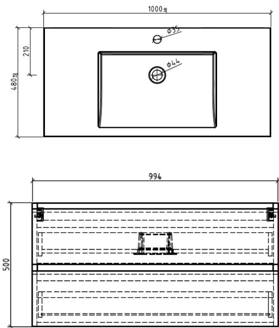
MUEBLE CITY 1000
