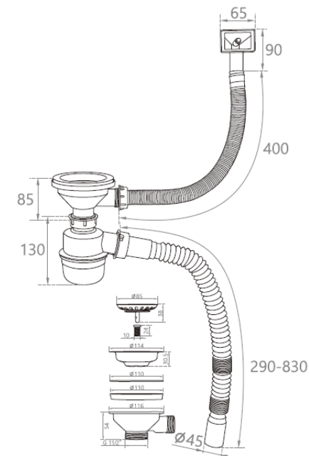
Detalle Técnico Desagüe LVP-09-0109
