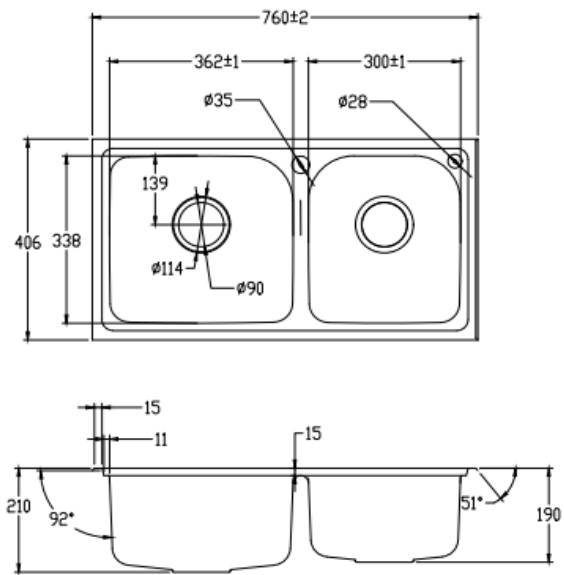
DETALLE TÉCNICO
