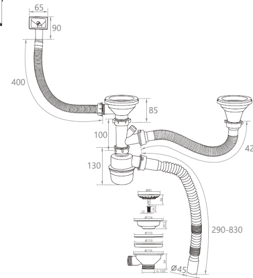
Detalle Técnico Desagüe LVP-09-0107
