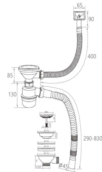
Detalle Técnico Desagüe LVP-09-0109
