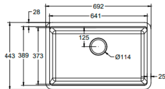
DETALLE TÉCNICO
