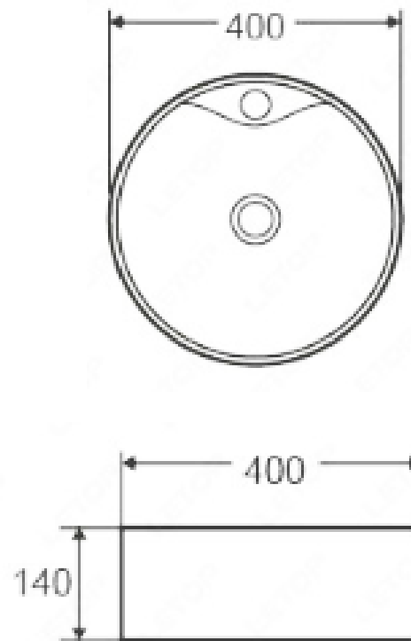
DETALLE TÉCNICO
