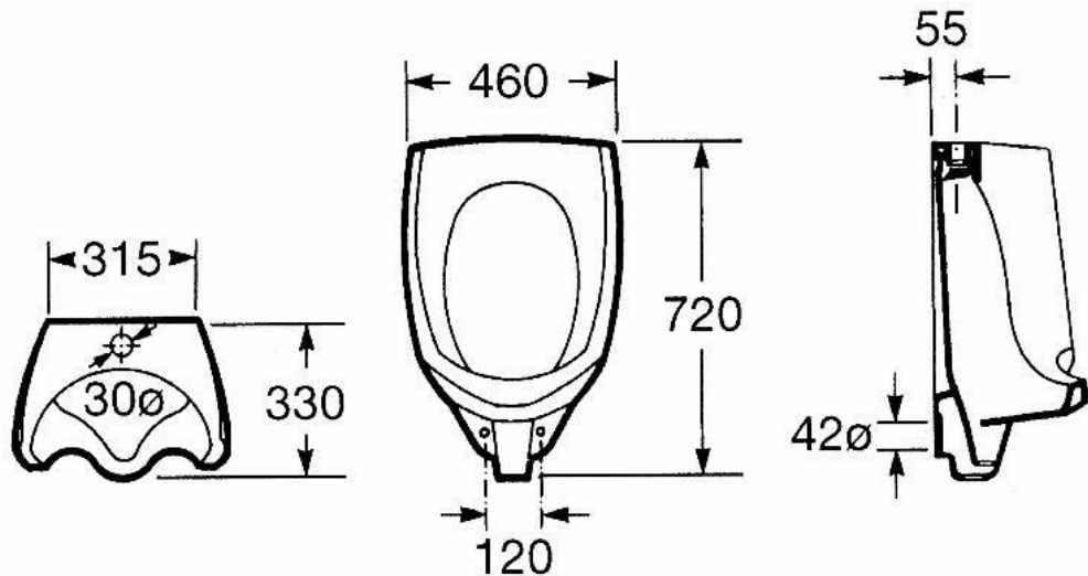
DETALLE TECNICO
