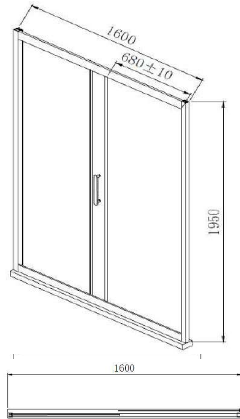
Dibujo técnico Anchura 1600 mm
