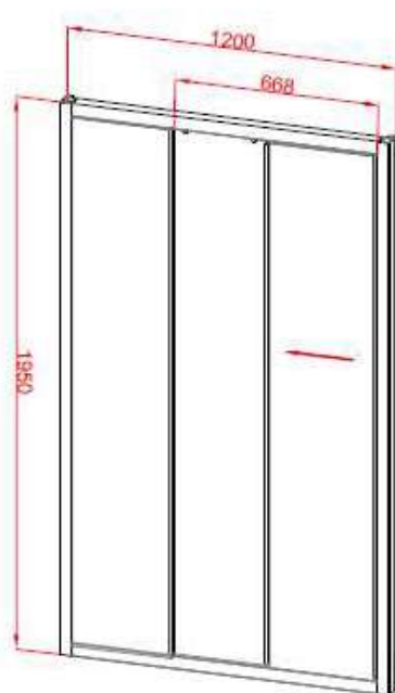
Dibujo técnico Anchura 1200 mm
