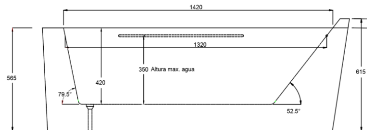
DETALLE TÉCNICO MEDIDAS EN MM
