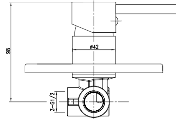
DETALLE TÉCNICO
