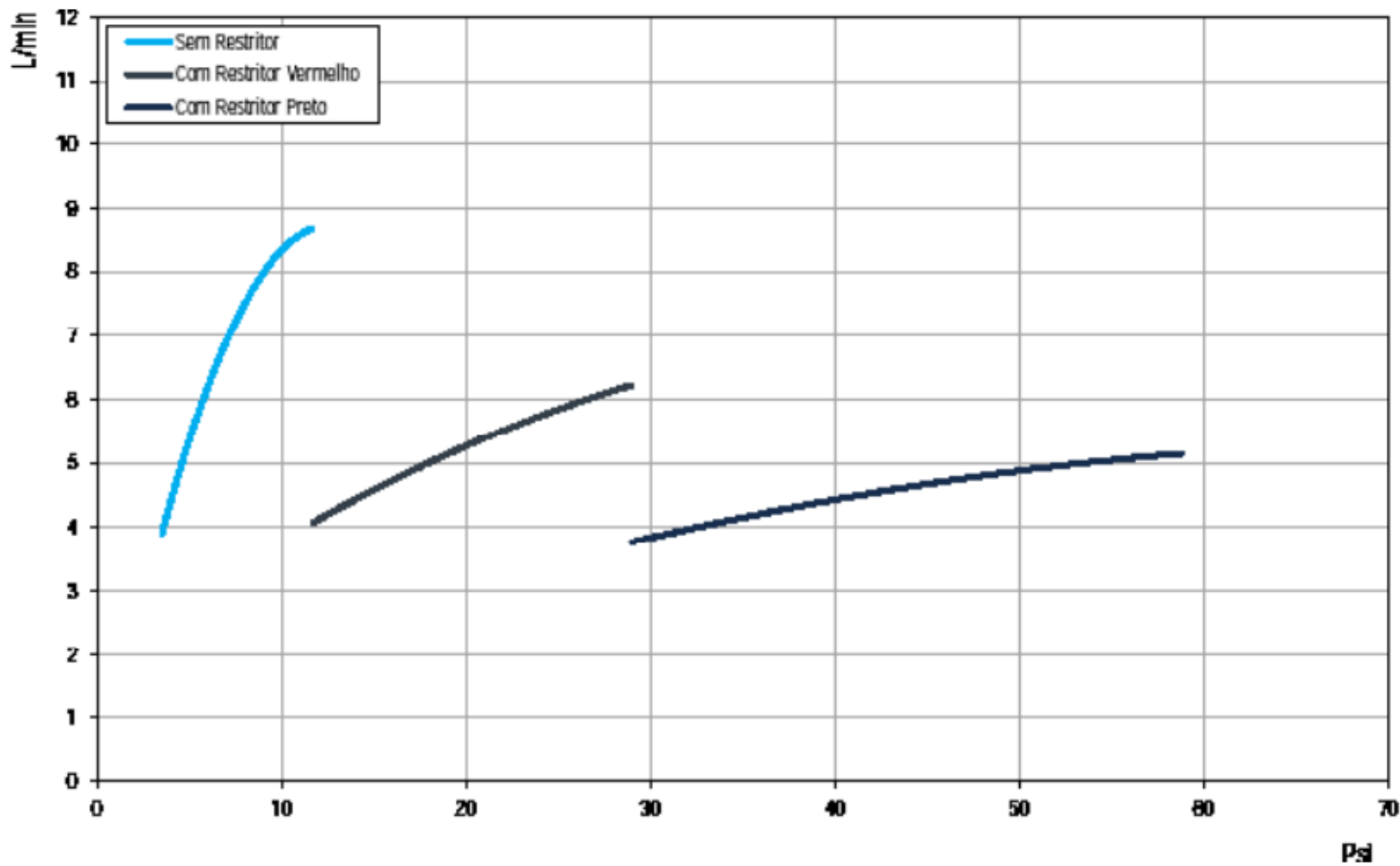
CURVA DE CAUDAL
