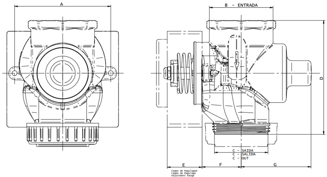
DETALLE TECNICO
