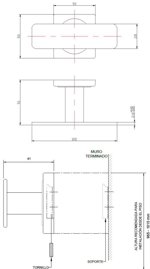
DIBUJO TÉCNICO MEDIDAS EN MM
