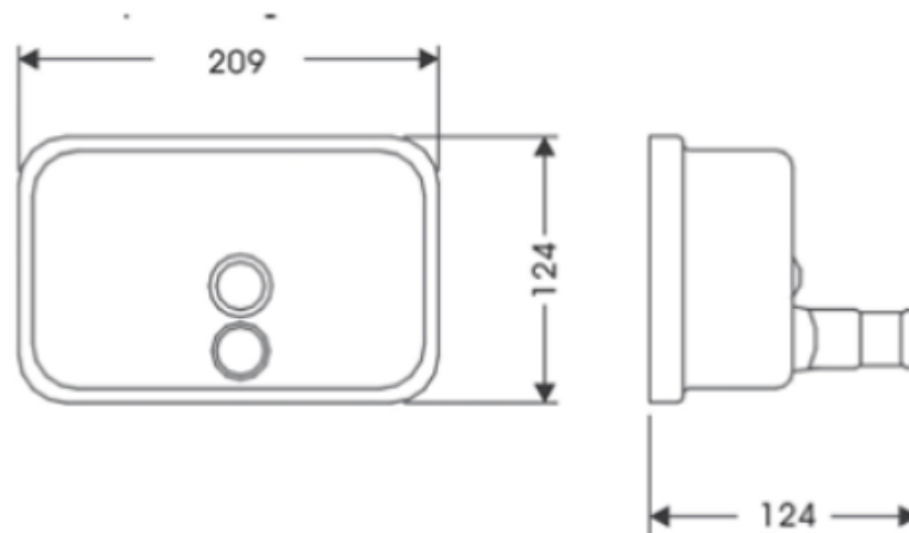
DETALLE TECNICO
